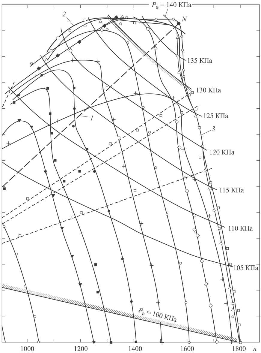
Рис. 4. Экспериментальная параметрическая зависимость крутящего момента от частоты вращения вала M(n) дизеля с турбонаддувом Д6Н с кривыми постоянного давления надвучного воздуха (обозначения см. рис. 2)
