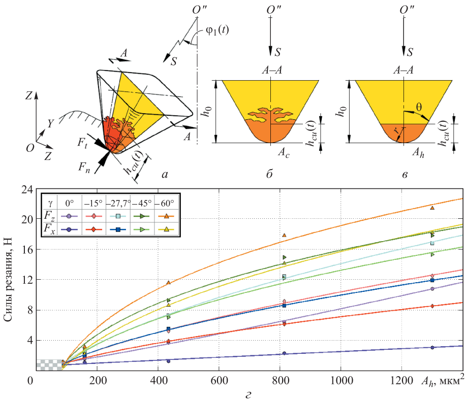
Рис. 7. Схема преобразования зерна в динамической модели (а); определение площади поперечного сечения контакта зерна и материала A_c (б), площади взрезания A_h (в); зависимость сил резания от площади поперечного сечения A_h при h_{cut} \geq r_0 = 10 \text{ мкм} (з)
