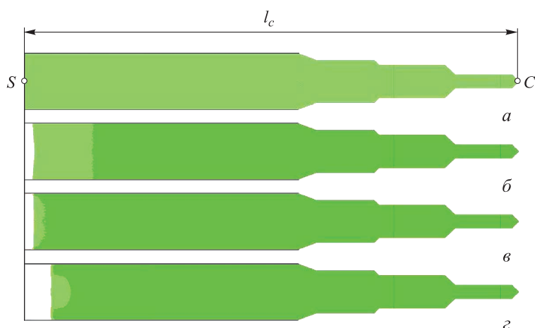
Рис. 4. Исходное состояние снаряжения с пределом текучести 5 МПа ( а ) и его осадка под действием осевой перегрузки, испытываемой ударником в процессе проникания, при использовании в расчетах модельных уравнений сжимаемости снаряжения УрС1 ( б ), УрС2 ( в ) и УрС3 ( г )
