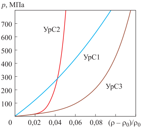
Рис. 2. Сравнительный анализ различных модельных вариантов баротропных зависимостей в форме Тэта, используемых для описания сжимаемости снаряжения
