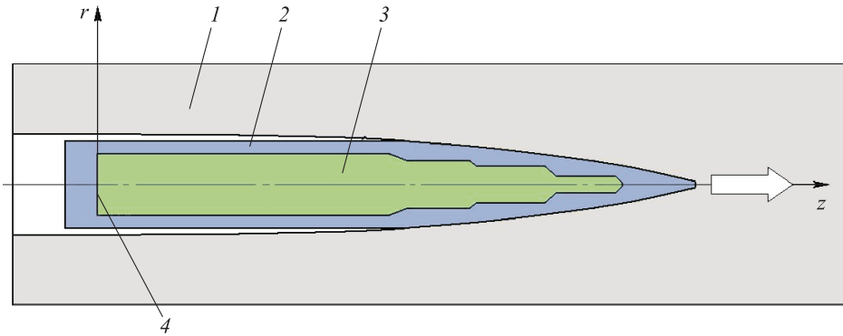
Рис. 1. Схема проникновения в бетонную преграду ударника со снаряжением:
