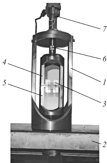
Рис. 3. Вертикальное нагрузочное устройство:
