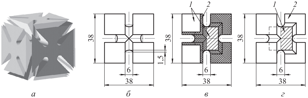
Рис. 7. Варианты конструкции образца для трехосного растяжения
