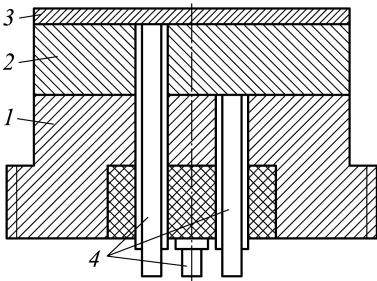
Рис. 1. Датчик теплового потока: 1 — корпус; 2 — теплотметрический элемент (дополнительная стенка); 3 — защитный слой; 4 — электроды
