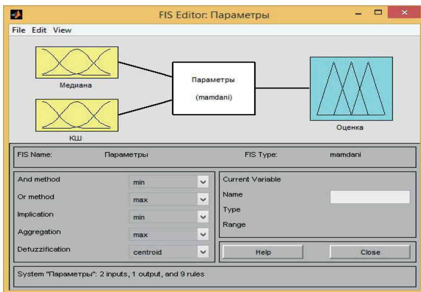
Рис. 1. Система для оценки качества деталей при варьировании зернистости кругов
