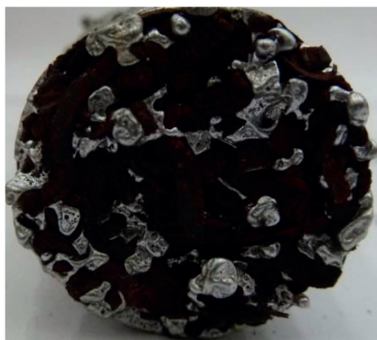
Рис. 3. Кристаллизация фронта горения расплава в канале вторичного окислителя
